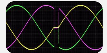
1ms ZVRT
